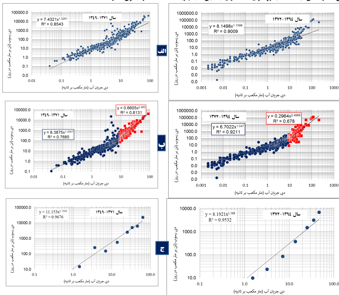
شکل ۳. منحنی سنجۀ (الف) یک‌خطی؛ (ب) دوخطی و (ج) حد وسط ایستگاه هیدرومتری اسکندری در دو دوره آماری براساس روش USBR
