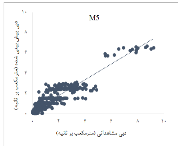
شکل ۲. نمودار پراکنش بین دبی مشاهداتی و پیش‌بینی شده فصل زمستان با روش M5
