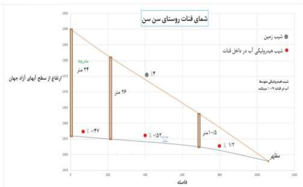
شکل ۴. شمای کلی و ترسیم دقیق نسبی قنات سن سن
