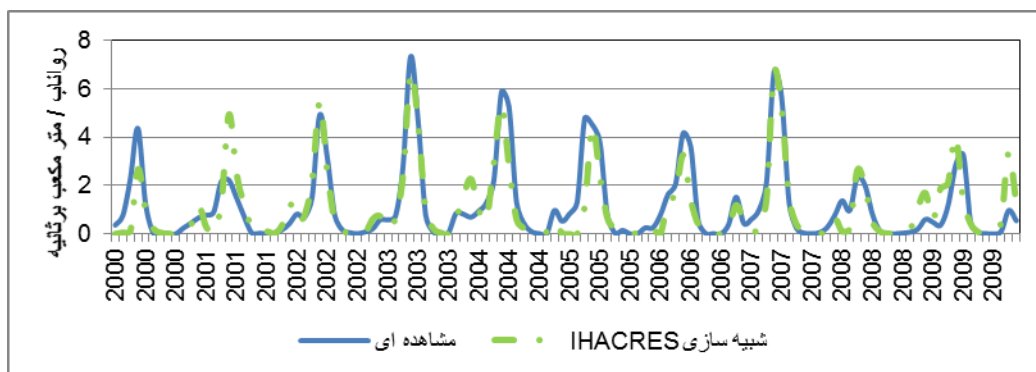
شکل ۱۱. شبیه‌سازی جریان ماهانه حوضه سد اکباتان در دوره صحت‌سنجی توسط مدل IHACRES
