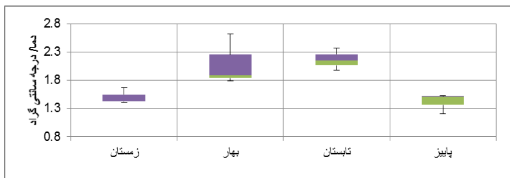
شکل ۸. باکس پلات تغییرات دمای فصلی منطقه تحت سناریوی A2، دوره ۲۰۴۵-۲۰۶۵ حوضه سد اکباتان
