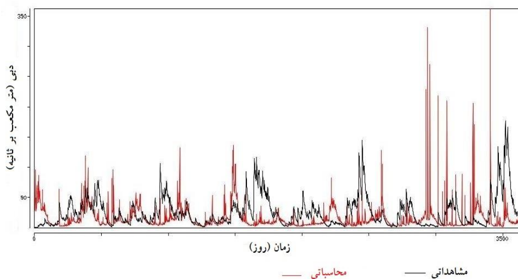
شکل ۶. مقایسه مقادیر جریان مشاهداتی و محاسباتی در مرحله ارزیابی مدل IHACRES رودخانه پلرود
