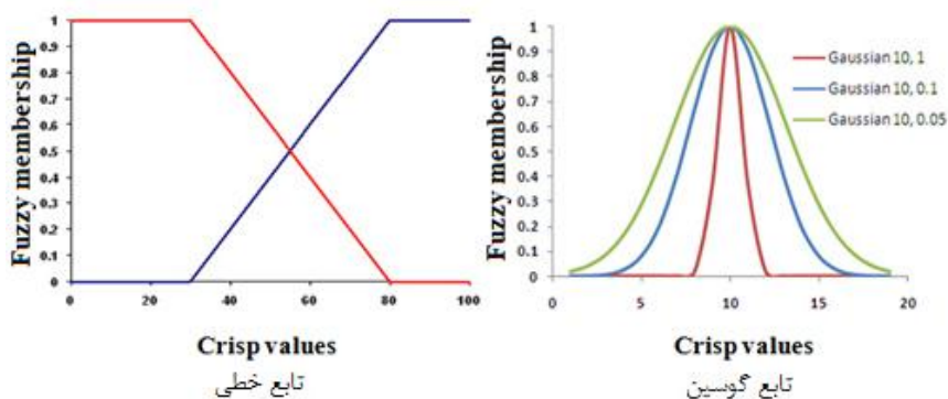
شکل ۱۱. توابع فازی [۱۷].
