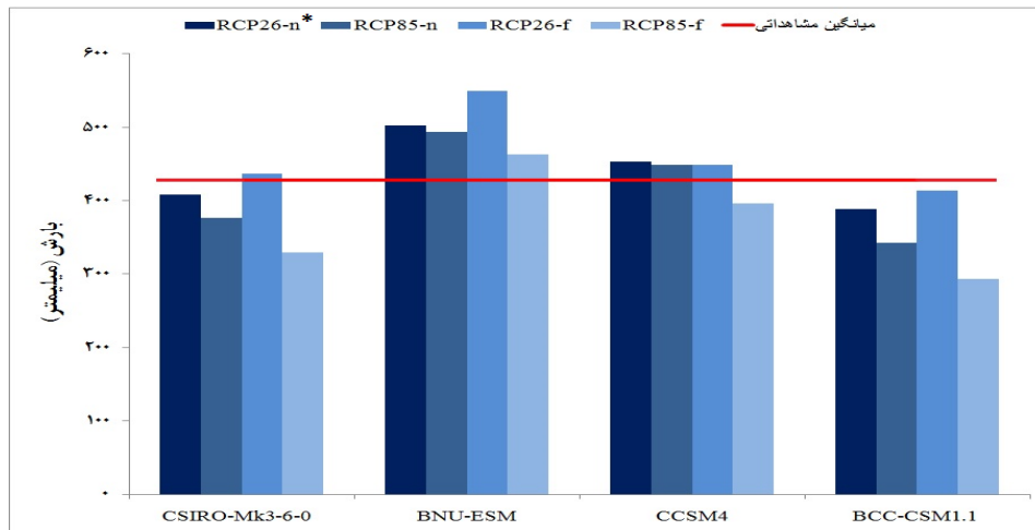
شکل ۳. تغییرات آبی میانگین بارش سالانه نسبت به میانگین مشاهده‌ای بر اساس مدل‌های CMIP5 و سناریوهای انتخابی (ایستگاه آران) *منظور از n آینده نزدیک و f آینده دور است.
