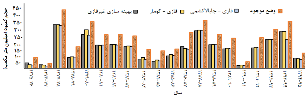
شکل ۱۳. حجم کمبود سالانه آب به روش کومار، جایالاکیشمی و بهینه‌سازی غیر فازی
