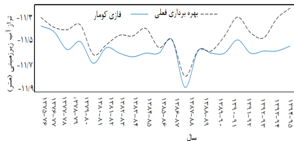
شکل ۱۱. تغییرات تراز آب زیرزمینی در بهره‌برداری فعلی و بهره‌برداری تلفیقی (روش کومار)
