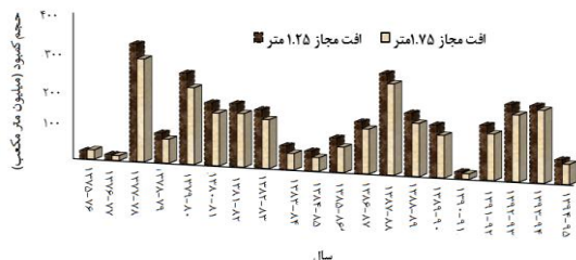
شکل ۱۵. حجم کمبود تأمین آب سالانه در تحلیل حساسیت افت سطح آب زیرزمینی (روش جایالاکیشمی)
