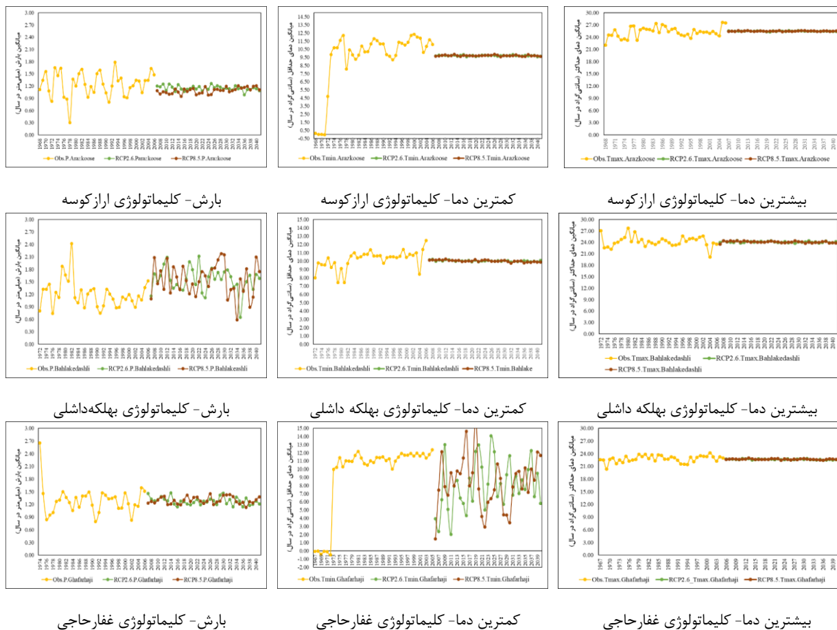
ادامه شکل ۵. روند تغییرات بارش، کمترین دما و بیشترین دما در دوره تاریخی و دوره ۲۰۰۶-۲۰۴۱ تحت سناریوهای RCP2.6 و RCP8.5 در حوضه رودخانه گرگان‌رود
