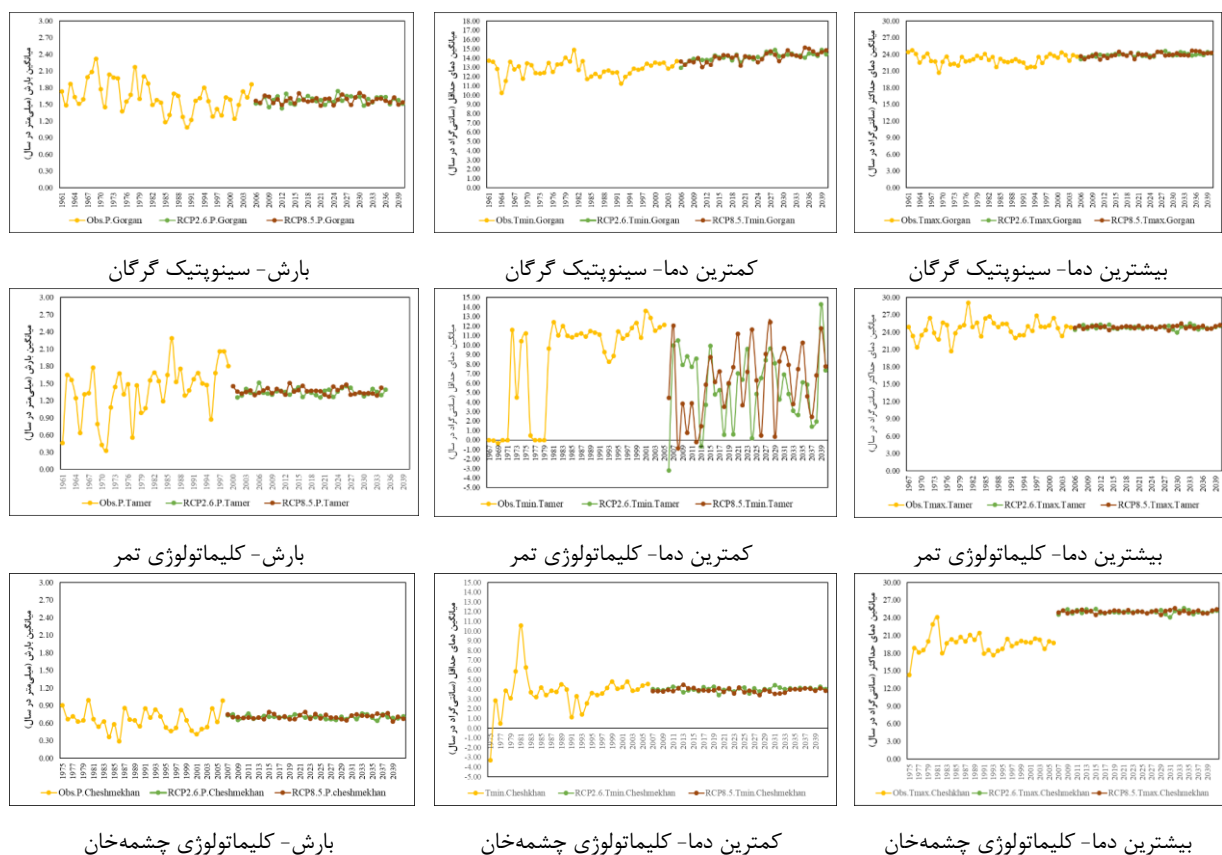
شکل ۵. روند تغییرات بارش، کمترین دما و بیشترین دما در دوره تاریخی و دوره ۲۰۰۶-۲۰۴۱ تحت سناریوهای RCP2.6 و RCP8.5 در حوضه رودخانه گرگان رود
