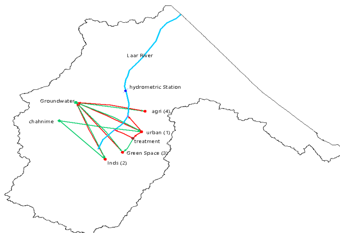
شکل ۲. شماتیک مدل WEAP در سناریوی مرجع
