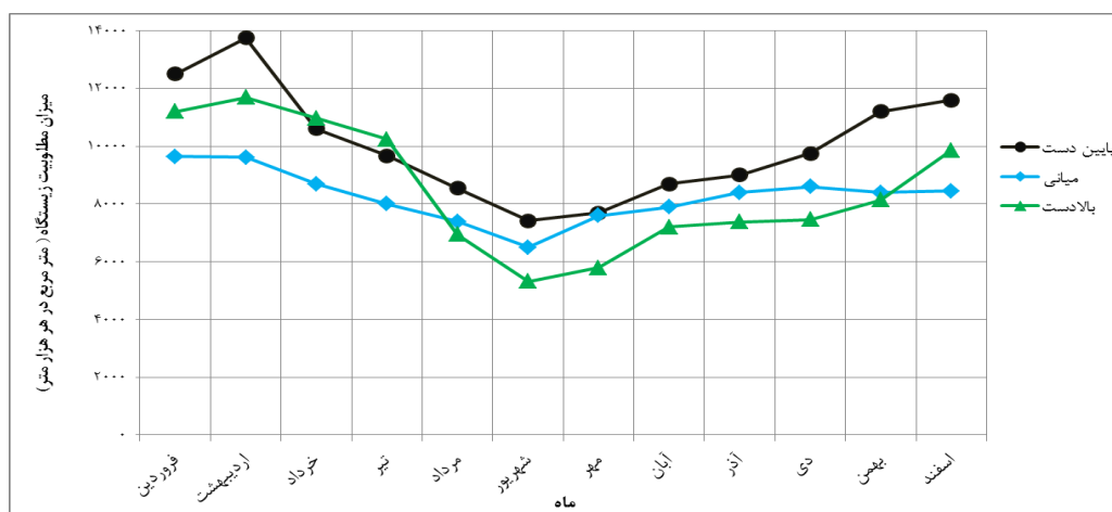
شکل ۸. منحنی سری زمانی میزان مطلوبیت زیستگاهی سیاه‌ماهی در بازه‌های مختلف رودخانه قره‌سو
