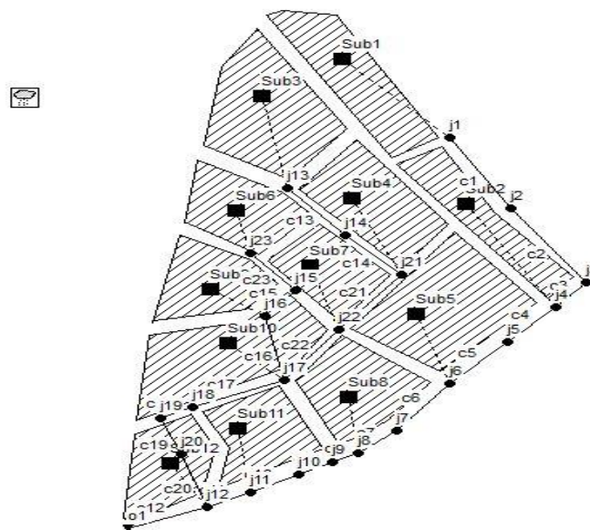
شکل ۳. مدل ساخته‌شده در نرم‌افزار SWMM
