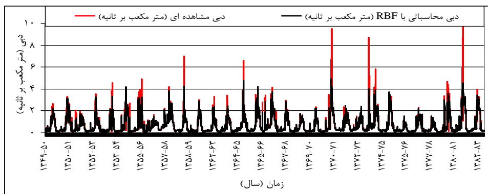
شکل ۴. نمودار دبی روزانه مشاهده‌ای و پیش‌بینی‌شده به روش RBF حوضه آبخیز امامه بر حسب ساختار ۵۴ برای سال‌های ۱۳۴۹-۱۳۵۰ تا ۱۳۸۳-۱۳۸۲ (آموزش)
