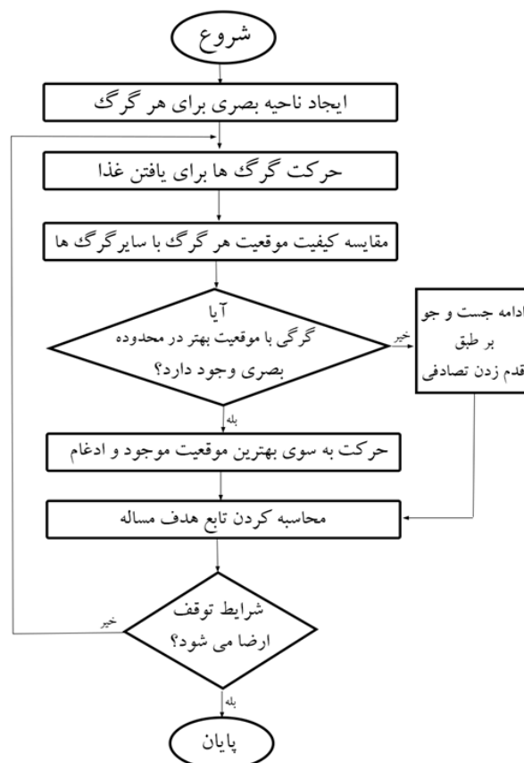
شکل ۳. فلوجارت الگوریتم جست و جوی گرگ
