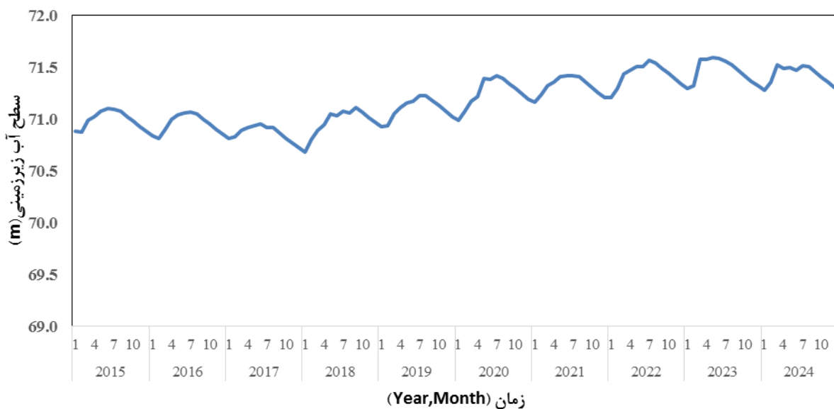
شکل ۸. هیدروگراف آب زیرزمینی آبخوان در سناریوی پنجم (تغییر اقلیم با سطح ریسک ۰/۹۰)
