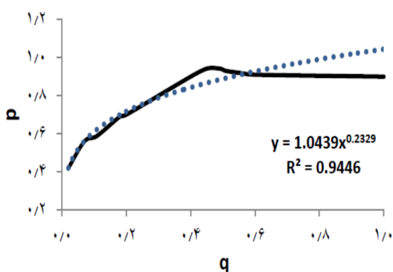
شکل ۴. مقطع عرضی سفیدرود به همراه منحنی بی بعد تغییرات محیط خیس شده در مقابل دبی
