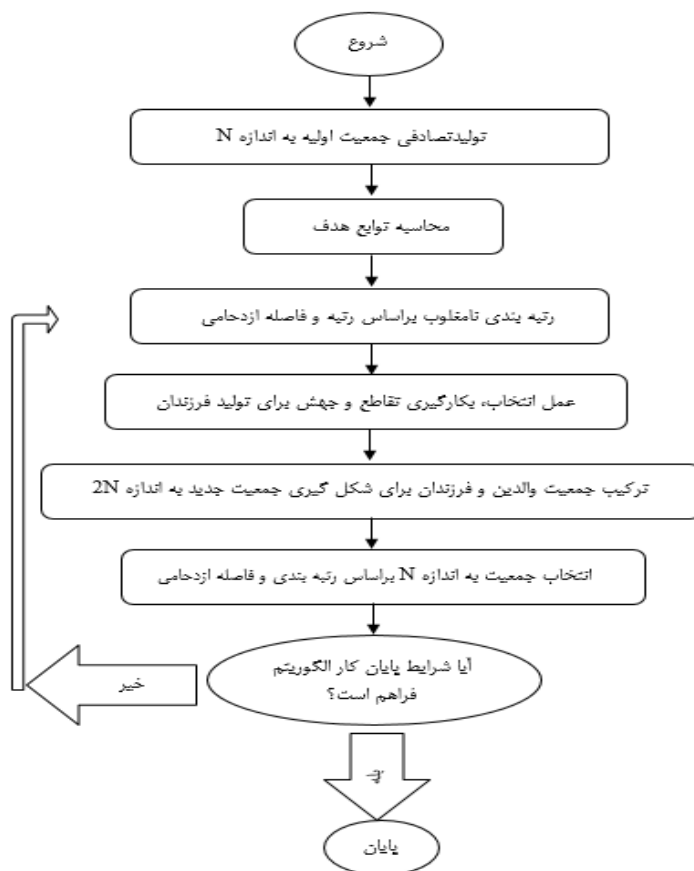
شکل ۲. چگونگی کار الگوریتم ژنتیک رتبه‌بندی نامغلوب (NSGA-II) (امین‌زاده و همکاران، ۱۳۹۵)
