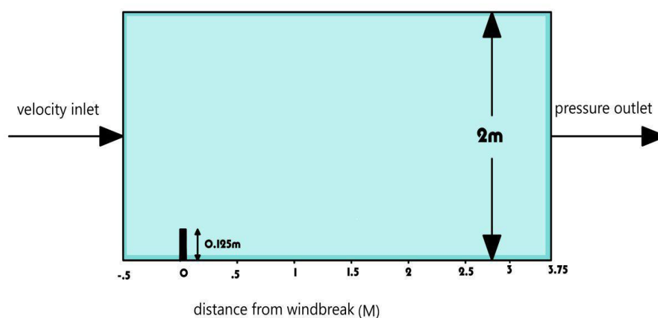
شکل ۳. محدوده جریان و بادشکن صلب شبیه‌سازی شده در ANSYS FLUENT
