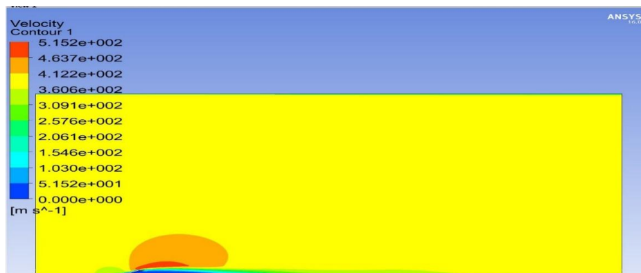
شکل ۶. پروفیل سرعت باد برای پنل خورشیدی (زاویه آزیموت 30^\circ و زاویه شیب 30^\circ درجه)
