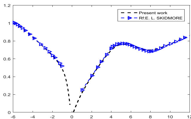
شکل ۵. مقایسه پروفیل سرعت باد بین تحقیق حاضر و اسکیمور و هاگن [۲۵]
