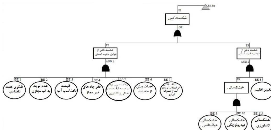
شکل ۴. درخت خطای حوضه دریاچه ارومیه - شکست کمی
