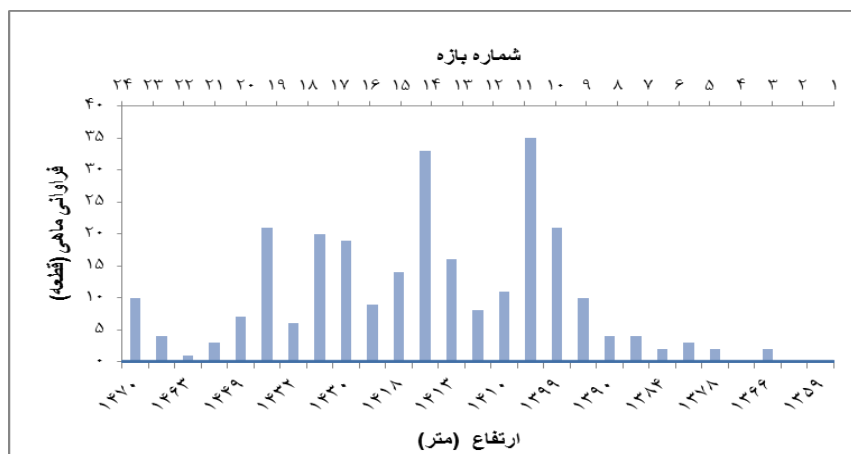
شکل ۳. تغییرات فراوانی سگ‌ماهی جویباری در طول رودخانه کردان
