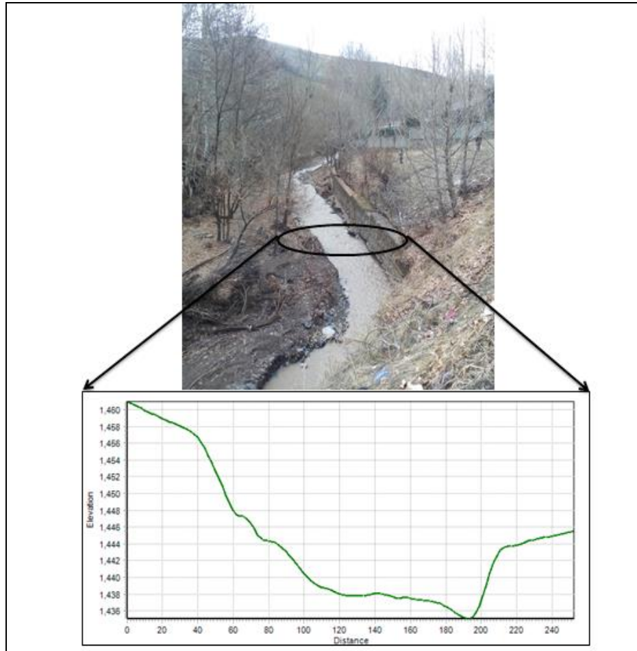
شکل ۲. نمایش مقطع عرضی در محیط نرم‌افزار GIS و انطباق آن با واقعیت (واقع در بازه ۲۴)
