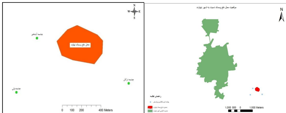
شکل ۲. موقعیت محل دفن پسماند نسبت به شهر نهاوند (راست) و موقعیت چشمه‌ها نسبت به محل دفن پسماند (چپ)
