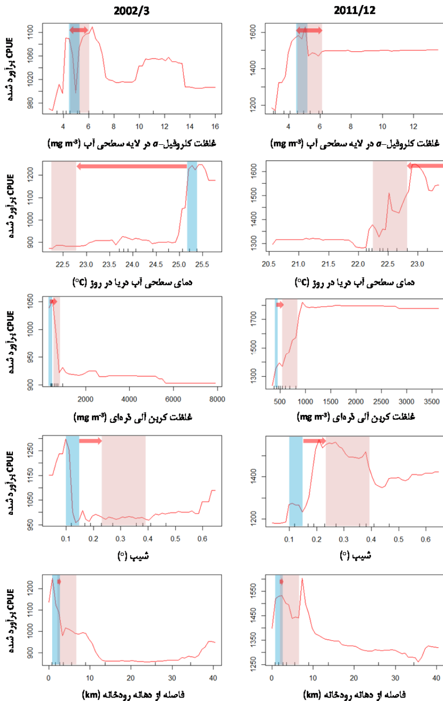
شکل ۲. نمودارهای وابستگی نسبی (pdp) و مقادیر بهینه از متغیرهای محیطی مورد بررسی در ارتباط با سطوح برآوردشده صید ماهی سفید (Estimated CPUE) در دوره‌های صید ۲۰۰۲/۳ و ۲۰۱۱/۱۲. کادراه‌های آبی رنگ و صورتی رنگ نشان‌دهنده بازه‌های بهینه متغیرهای محیطی برای ماهی به ترتیب در دوره‌های صید ۲۰۰۲/۳ و ۲۰۱۱/۱۲ هستند. فلش‌های قرمز رنگ تغییرات بازه‌های بهینه در طول دوره ۱۰ ساله را نشان می‌دهند.
