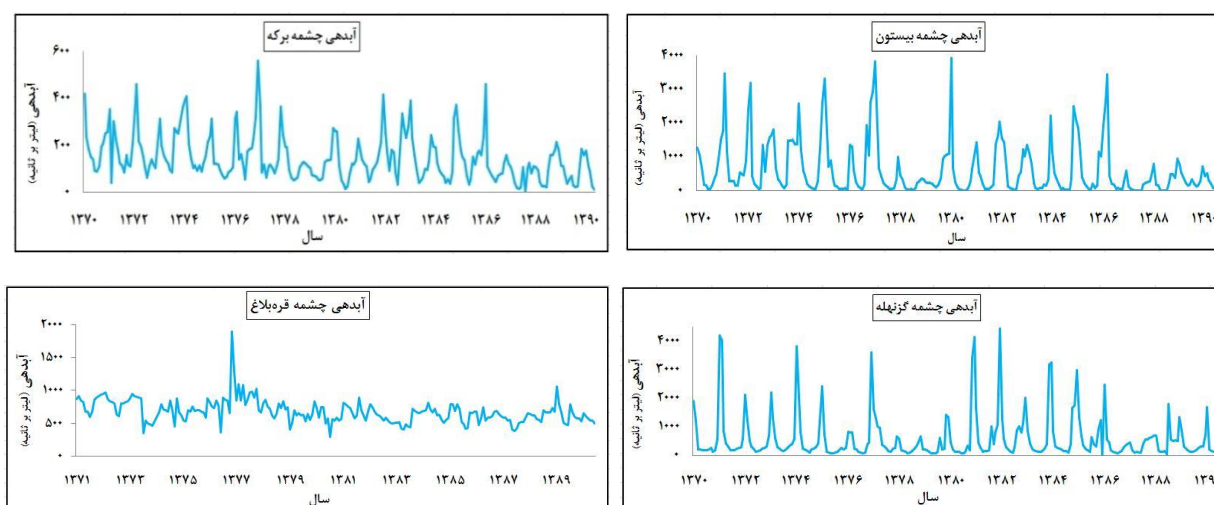
شکل ۴. تغییرات بلندمدت آبدهی چشمه‌های بیستون، برکه، گزنه‌له و قره‌بلاغ
