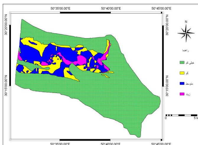
شکل ۶. نقشه پهنه‌بندی فرسایش خندقی به روش فازی گامی ۰/۵
