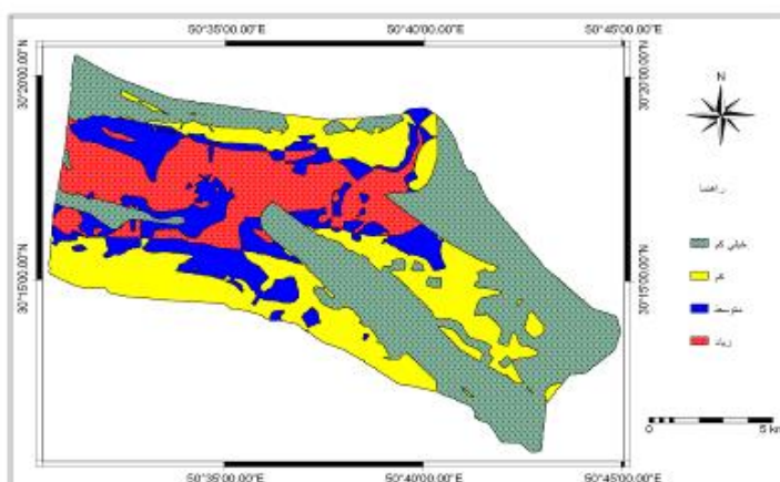
شکل ۷. نقشه پهنه‌بندی فرسایش خندقی به روش فازی گامی ۰/۸
