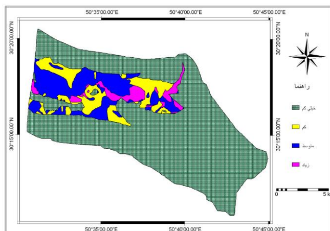
شکل ۵. نقشه پهنه‌بندی فرسایش خندقی به روش فازی گامی ۰/۲
