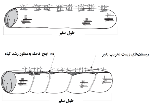
شکل ۱۷. نمایی از روش مهندسی زیستی Plant Roll
