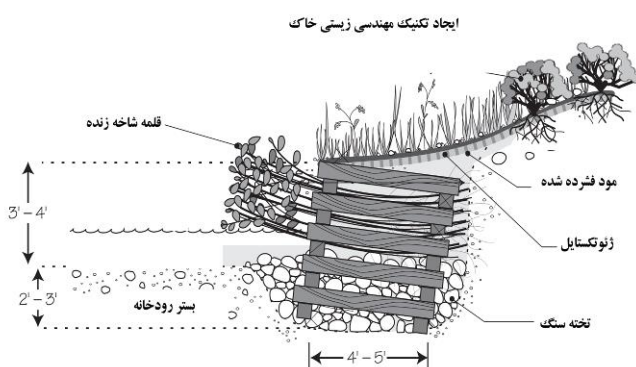
شکل ۲۶. نمایی از روش مهندسی زیستی Live Cribwall
