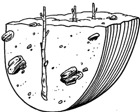
شکل ۵. نمایی از روش مهندسی زیستی Live Stacking
