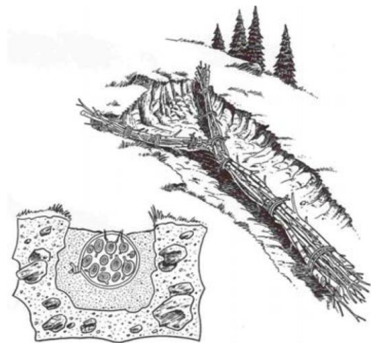
شکل ۱. نمایی از روش مهندسی زیستی Live Pole Drains
