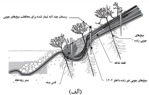
شکل ۸. نمایشی از روش مهندسی زیستی Brush Mattress (الف) و روش اجرای آن (ب)
