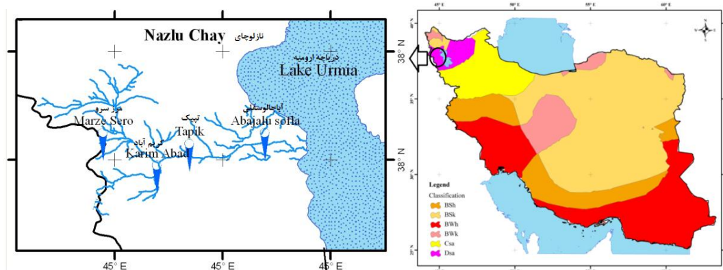
شکل ۱. موقعیت جغرافیایی حوضه آبریز نازلوچای و ایستگاه‌های هیدرومتری منتخب بر اساس طبقه‌بندی کوپن گیجر
