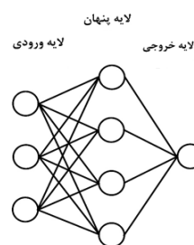
شکل ۲. ساختار شبکه عصبی پرسپترون چندلایه با یک لایه پنهان
