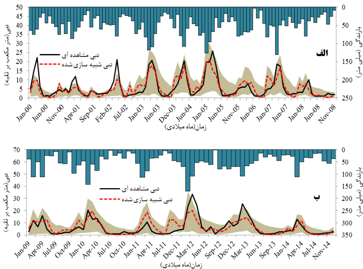
شکل ۴. سری زمانی منتخب دبی ماهانه شبیه‌سازی شده و مشاهداتی ایستگاه هیدرومتری آرازکوسه در مرحله واسنجی (الف) و صحت‌سنجی (ب)
